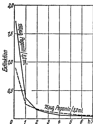
Abb. 3. Einfluß der Zeit nach dem Zusatz von Jodjodkalium-Reagens zu Peganinlösungen auf den Nachweis des Peganins
