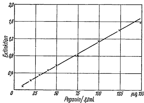
Abb. 2. Photometrischer Nachweis von Peganin mit Jodjodkalium-Reagens (Schichtdicke 1 cm; Wellenlänge 700 m \mu )
